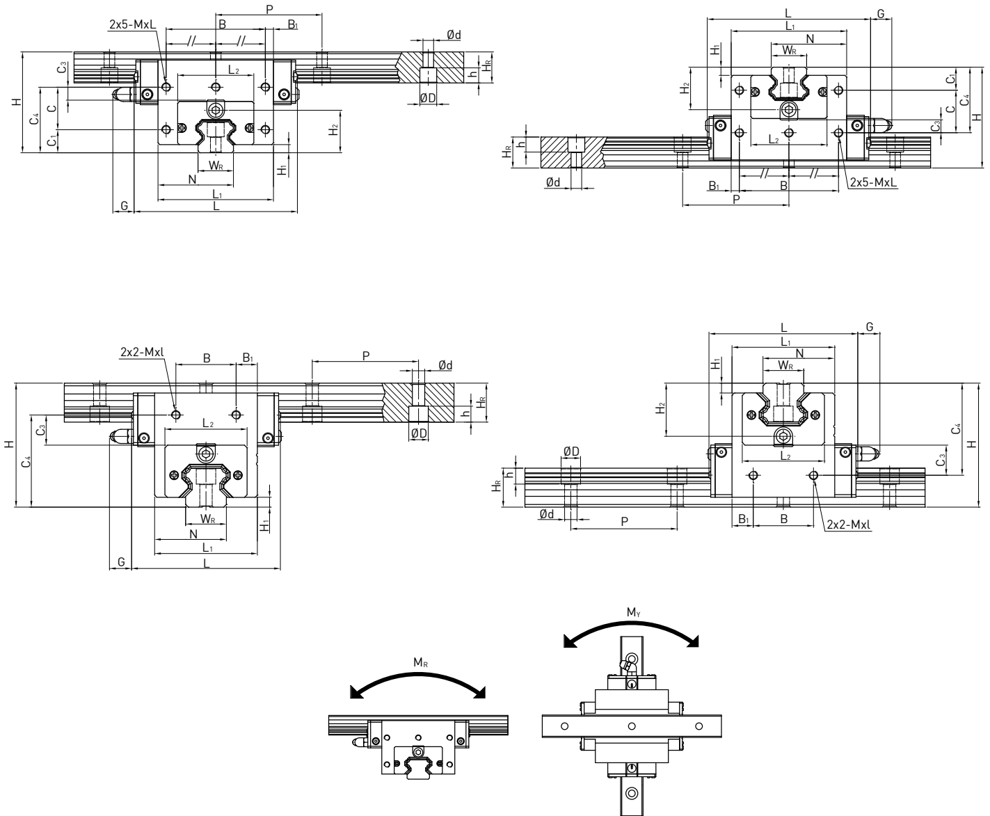
2-12-12 AG系列線性滑軌尺寸表
