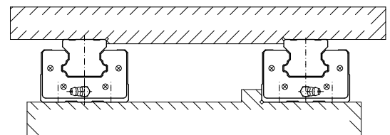
兩支滑軌滑塊移動配置
